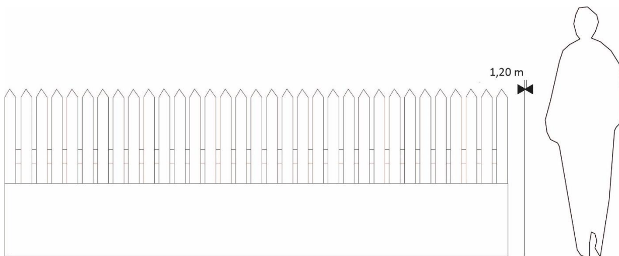
Dispositif à claire-voie supporté par un mur-bahut
